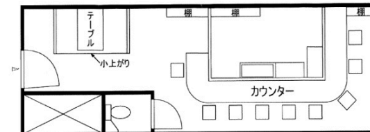
1階店舗 20.7㎡(6.26坪)
